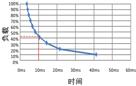
DDR-120A-12
